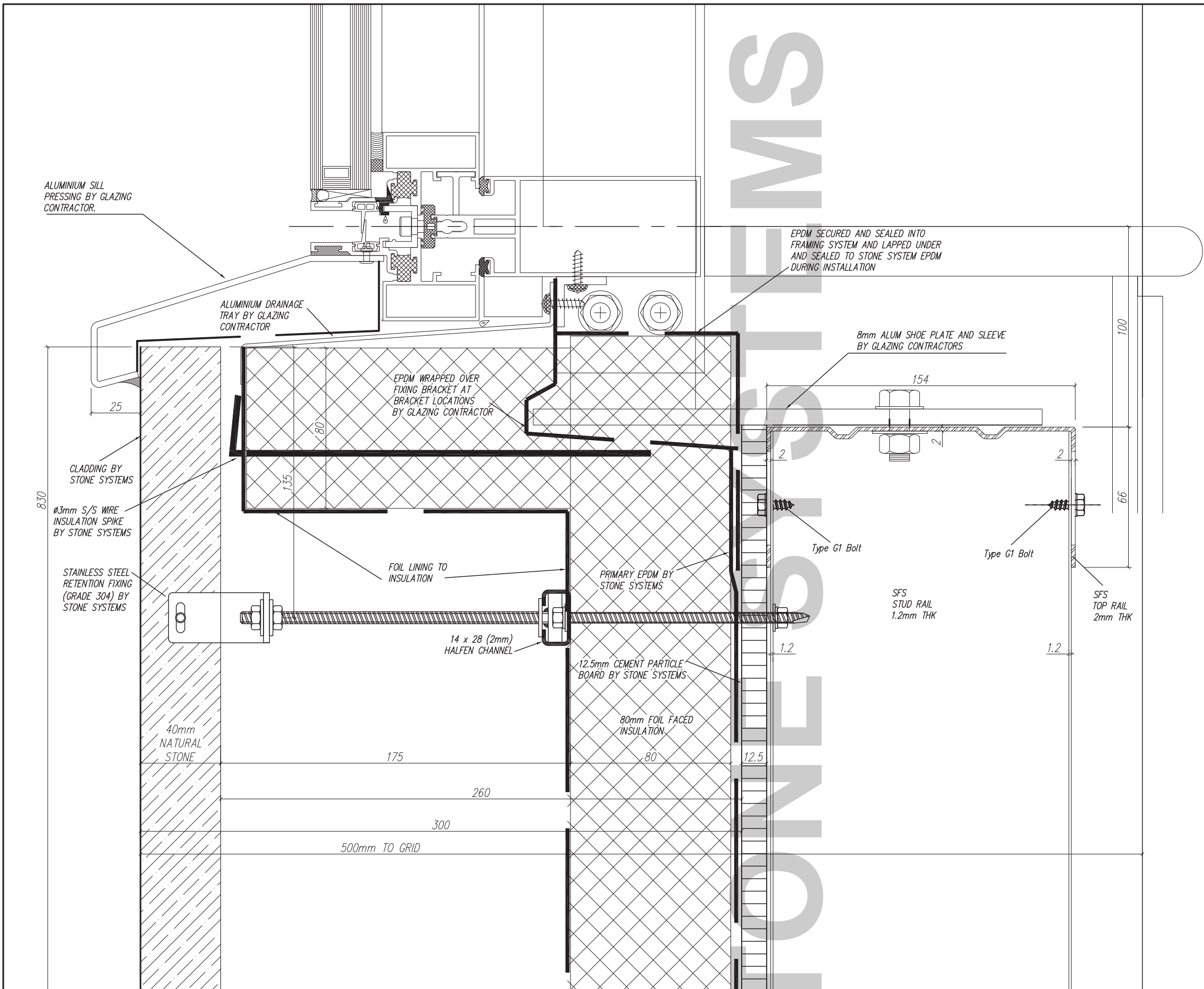
CILL DETAIL: SCALE: 1:2
