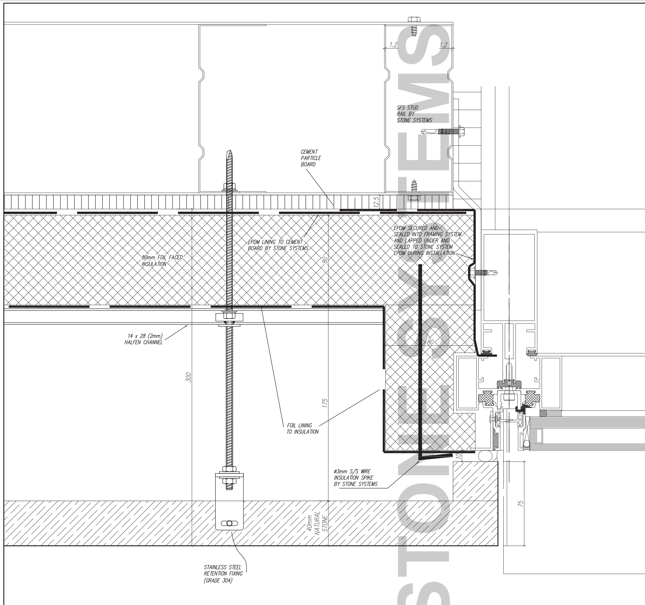
CILL DETAIL: SCALE: 1:2
