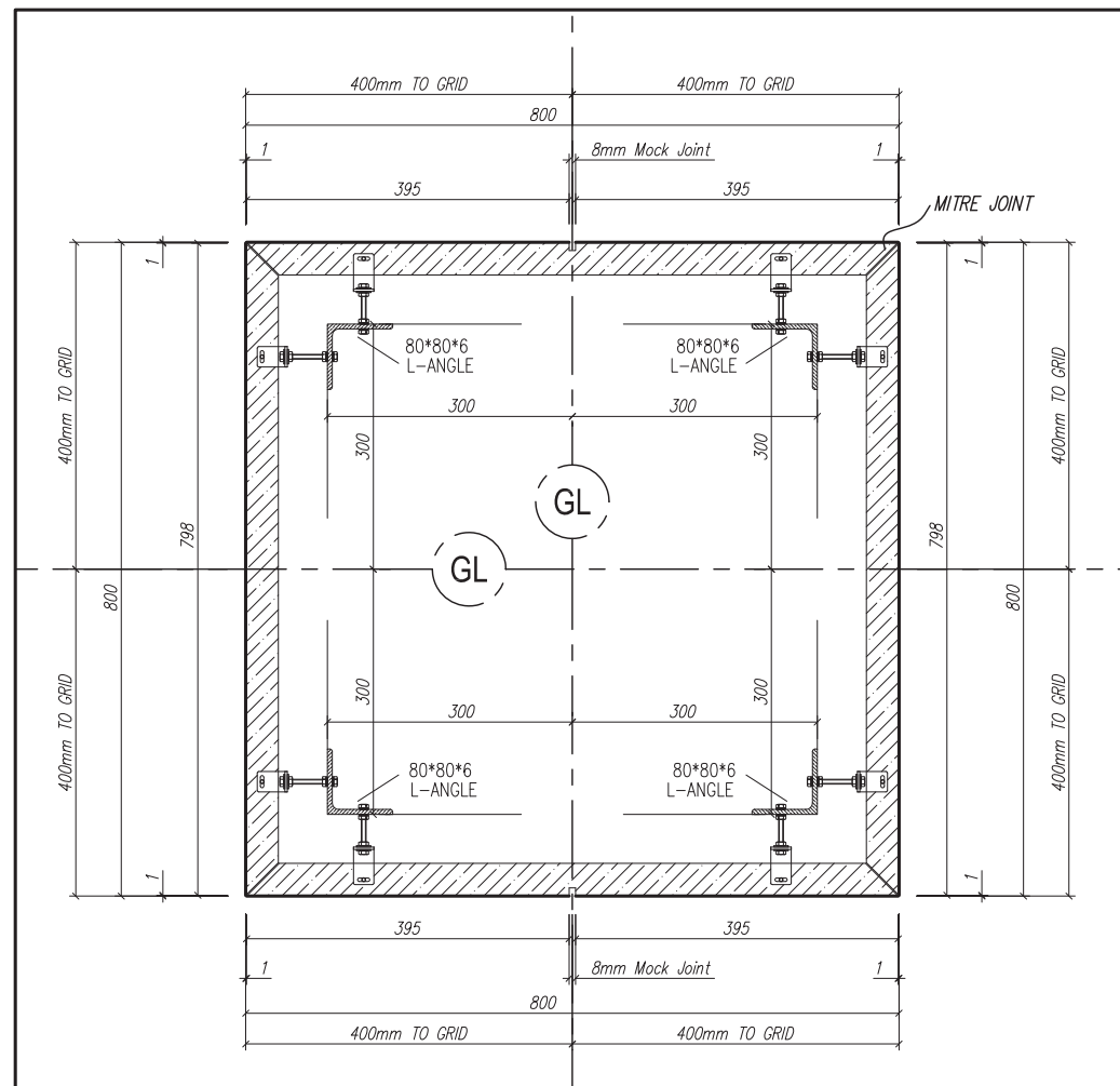
STEEL SUB COLUMN FRAME: SCALE: 1:10
