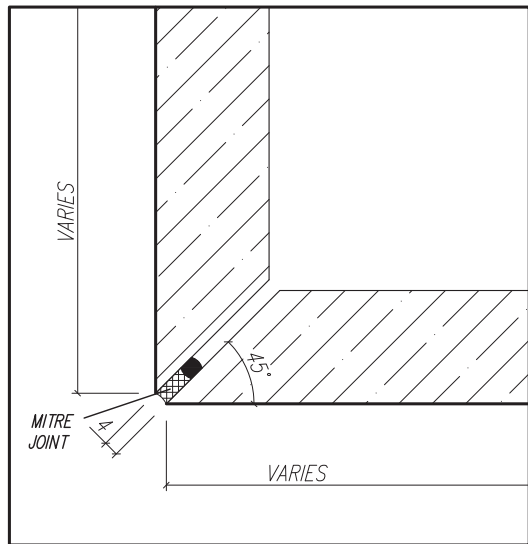
MITRE JOINT DETAIL: SCALE: 1:2
