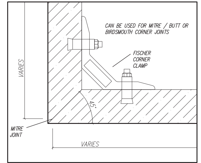
FISCHER CORNER CLAMP DETAIL: SCALE: 1:2
