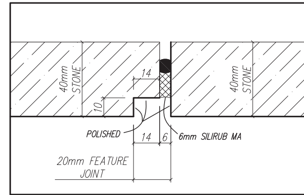
REBATE DETAIL: SCALE: 1:2
